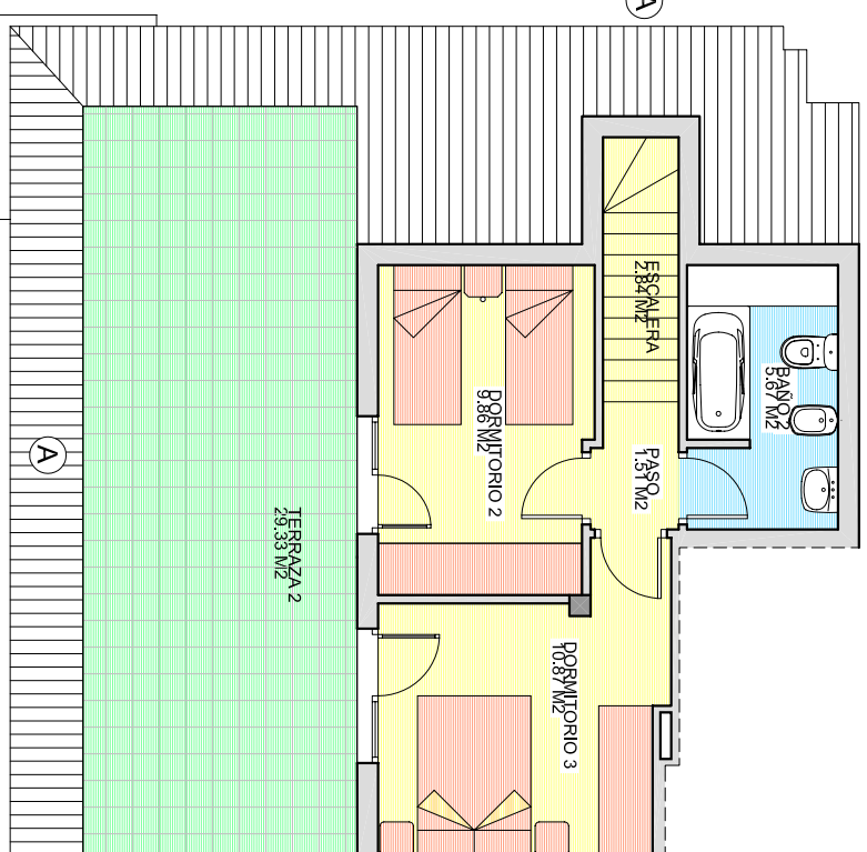
PLANTA CUBIERTA VIVIENDA A
