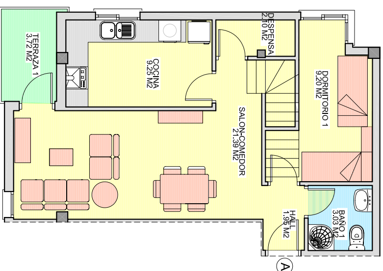
PLANTA SUPERIOR VIVIENDA A
