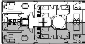
VIVIENDA B - PLANTA PRIMERA Y SEGUNDA
