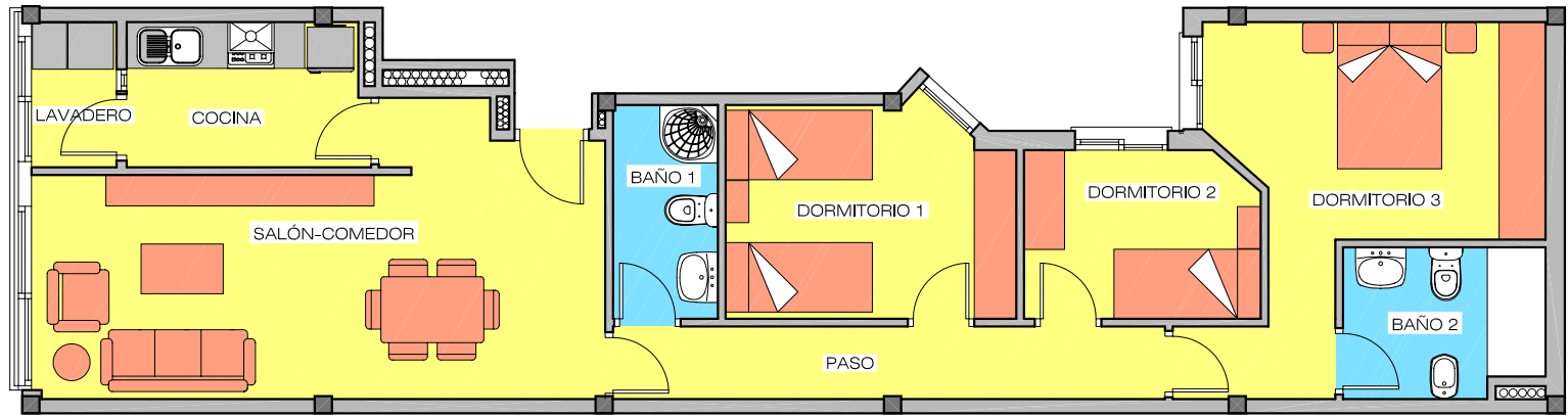
VIVIENDA B - PLANTA PRIMERA Y SEGUNDA
